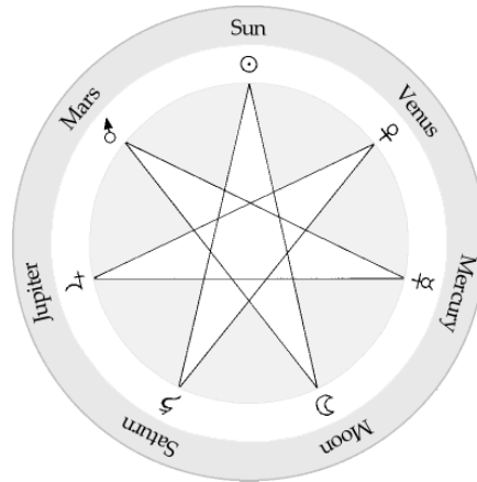
図 七芒星
