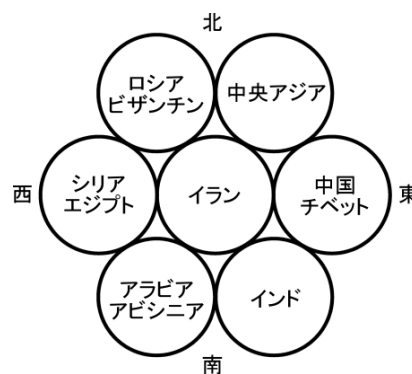
図2 後代の七州
