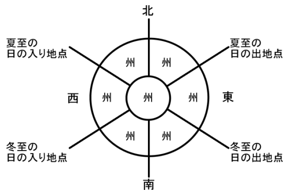
図1 七つの州
